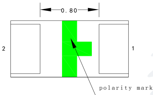
Fig.1-3 Bottom view 背面视图
